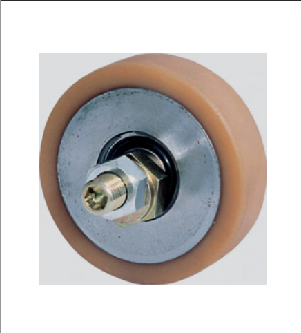
Aufzugsrolle mit Exzenter/ elevator roller with cam/ galet d'ascenseur avec excentrique
